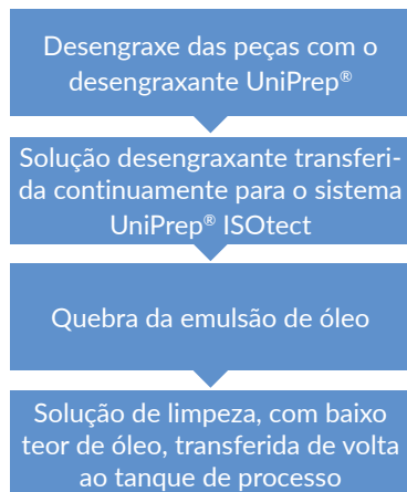
Fig. 2: Fluxo do processo com o UniPrep® ISOtect
